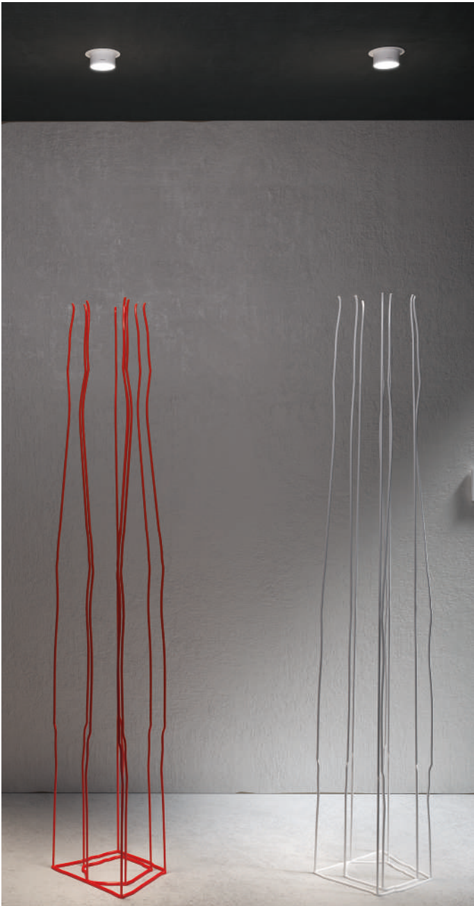
6w 350mA 840lm 3000K - 230V
