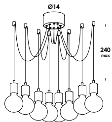
14/s8 dec. 8 E27 max 60w
