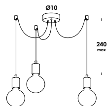
10/s3 dec. 3 E27 max 60w
