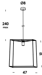
cubo 50/so E27 max 60w
