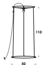
t.cono 50/ph on-off E27 max 60w
