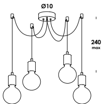
10/s4 dec. 4 E27 max 60w
