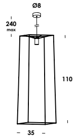
cubo 35/so 110 E27 max 60w
