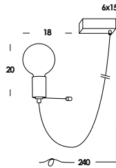
15/ap dec. E27 max 60w
