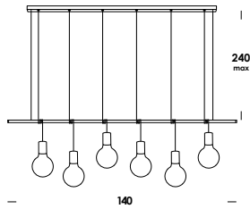
140/s6 6 E27 max 60w
