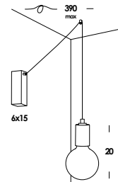
15/s2 dec. 2 E27 max 60w
