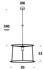
t.cono 50/so E27 max 60w
