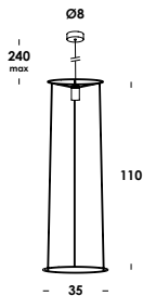
t.cono 35/so 110 E27 max 60w
