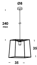
cubo 35/so E27 max 60w
