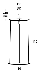
t.cono 50/so 110 E27 max 60w
