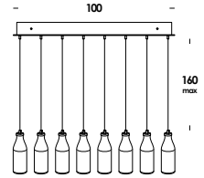
100/s8 8 E14 max 40w
