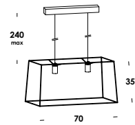
twin 70/s2 2 E27 max 60w
