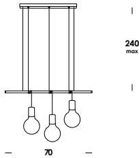
70/s3 3 E27 max 60w
