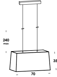
cocoon 70/so 2 E27 max 60w
