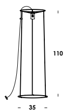
t.cono 35/ph on-off E27 max 60w
