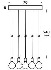
5up/so 5 E27 max 60w
