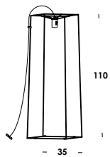
cubo 35/ph on-off E27 max 60w
