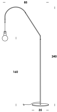
85/ph on/off E27 max 60w
