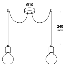
10/s2 dec. 2 E27 max 60w
